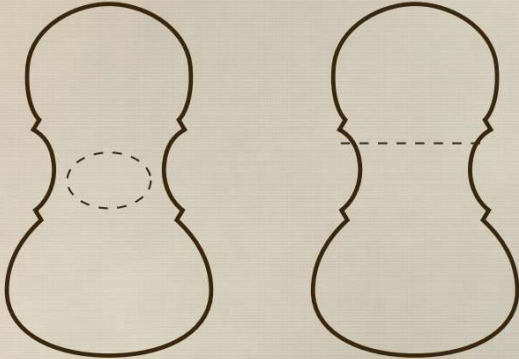
AO · 100 Hz Helmholtz air mode
